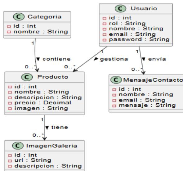
Diagrama de Datos / Estructura de Información
